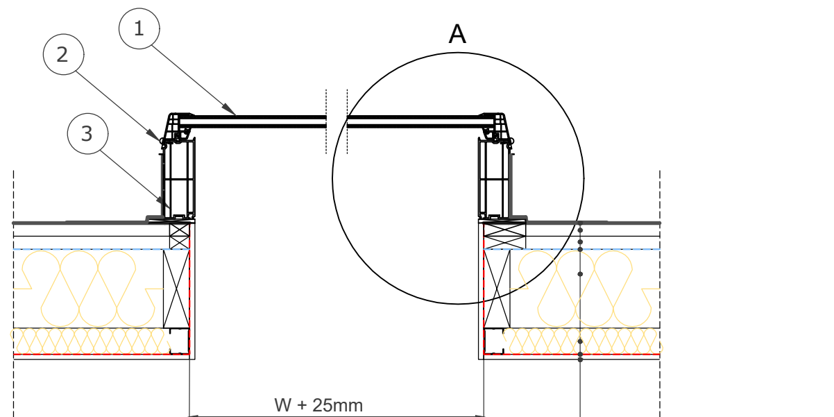
Section A-A' 1:10
