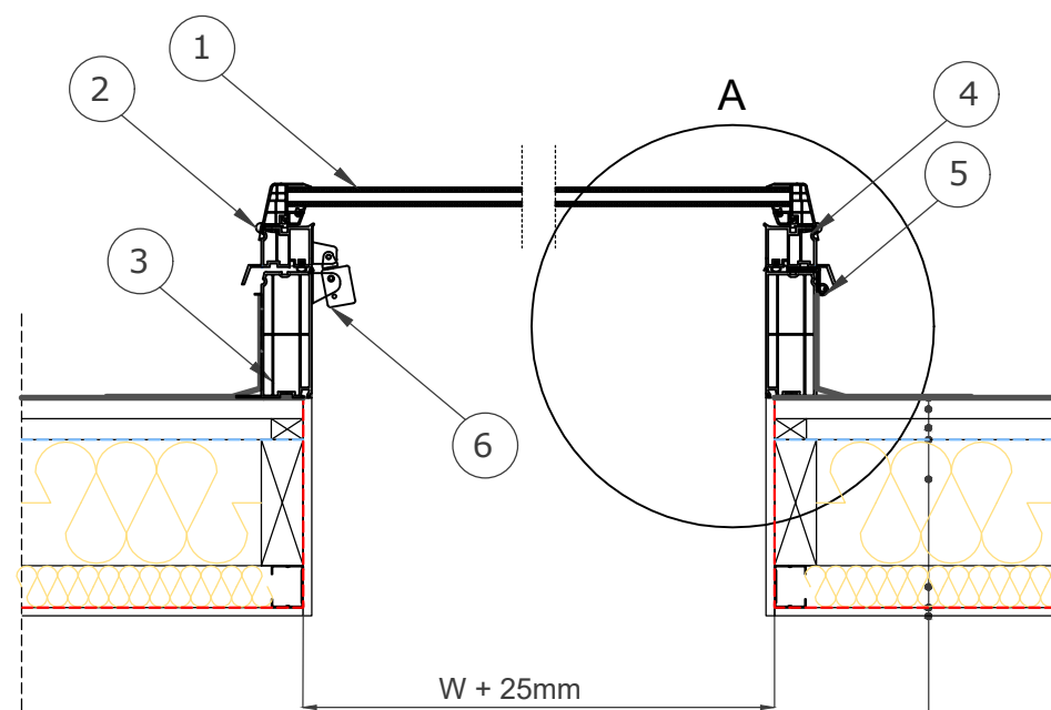
Section A-A' 1:10
