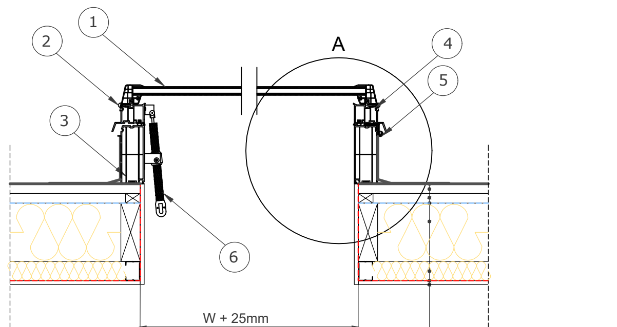
Section A-A' 1:10
