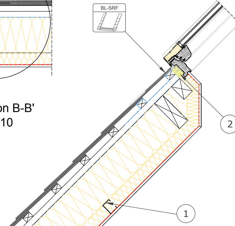
Section A-A' 1:10
