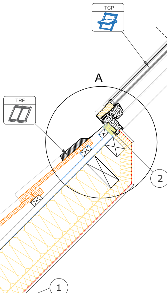
Section A-A' 1:10
