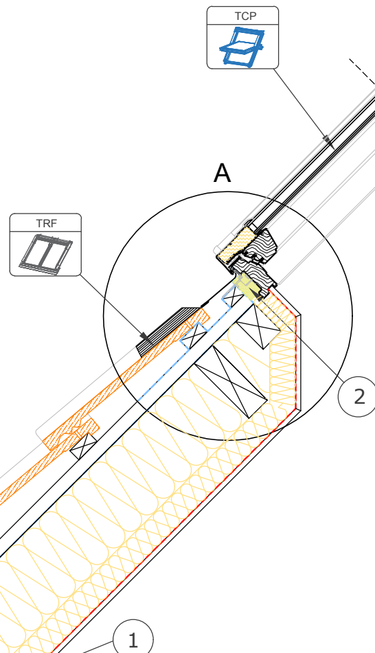
Section A-A' 1:10
